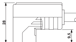
Ventilstecker, Bauform C, Seitenansicht
