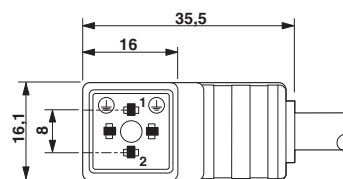
Maßzeichnung
