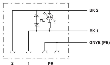
Kontaktbelegung des Ventilsteckers
