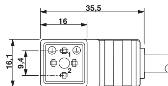
Maßzeichnung
