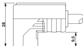
Ventilstecker, Bauform CI, Seitenansicht
