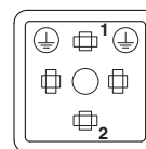
Polbild Ventilstecker, Bauform CI
