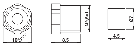
Maßzeichnung
