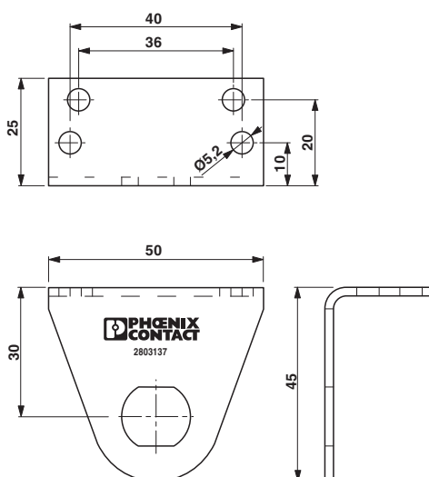
Maßzeichnung
