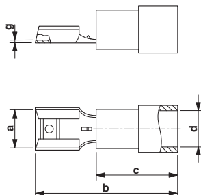
Maßzeichnung
