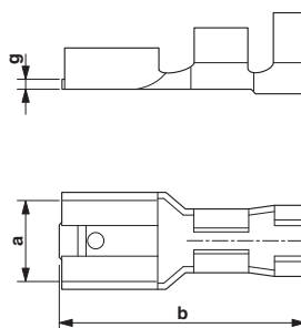
Maßzeichnung
