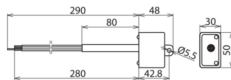
Maßbild DCOR L 3P 275 SO IP
