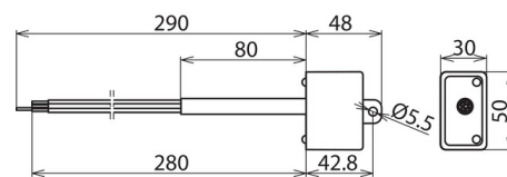
Maßbild DCOR L 2P 275 SO IP
