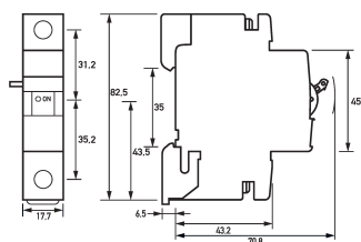
Maßzeichnung Gruppenansicht
