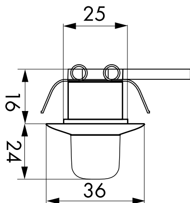
Bemaßung 92933
