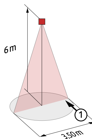
Reichweitendiagramm 1: Quer zum Melder gehen
