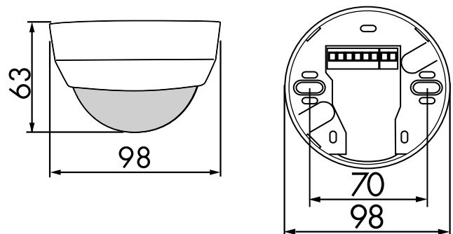
Bemaßung 92580
