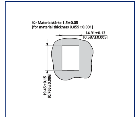
Einbauausschnitt
