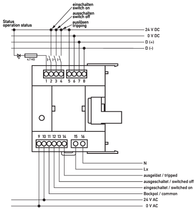
Anschlusschema
