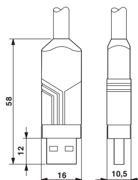
Maßzeichnung
