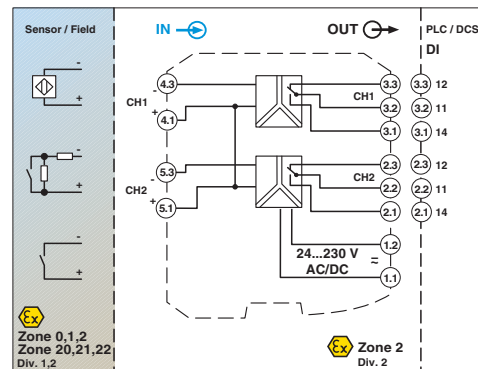
Blockschaltbild
