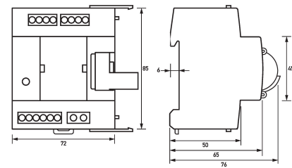
Maßzeichnung Gruppenansicht
