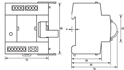
Maßzeichnung Gruppenansicht
