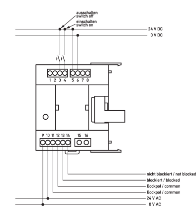
Anschlusschema
