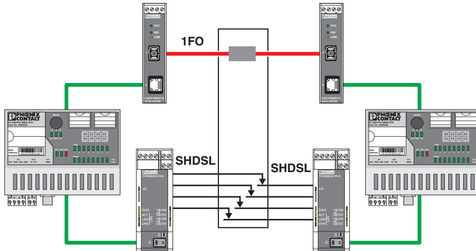
Redundante Schleifringkommunikation
