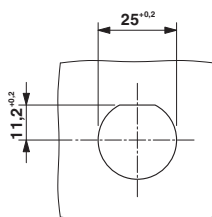
Maßzeichnung
