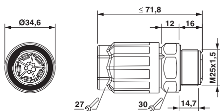
Maßzeichnung QPD W 4PE2,5 M25
