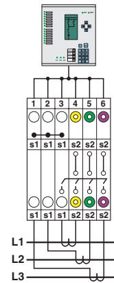
Verketteter Drei-Phasen-Stromwandlersatz
