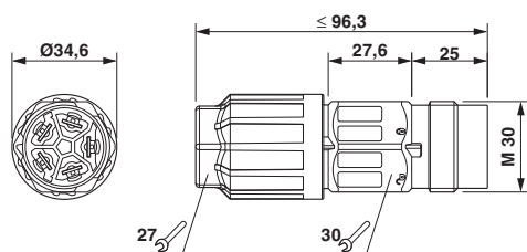
Maßzeichnung QPD C 5x2,5
