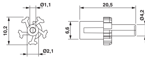
Maßzeichnung
