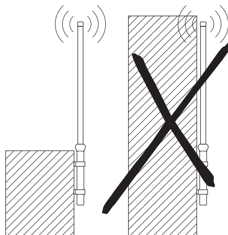
Schemazeichnung
