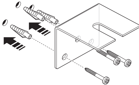
Schemazeichnung
