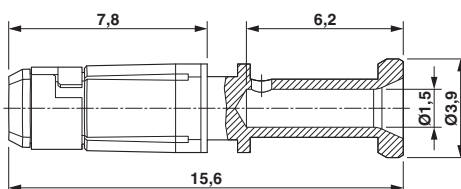
Maßzeichnung
