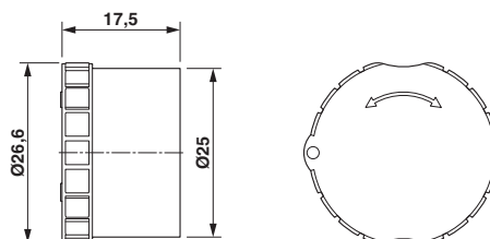
Maßzeichnung
