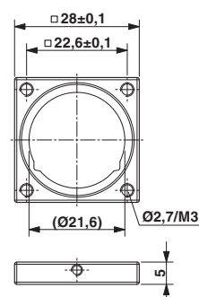
Maßzeichnung
