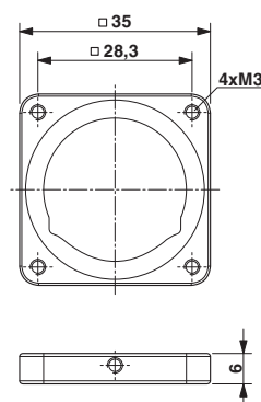
Maßzeichnung
