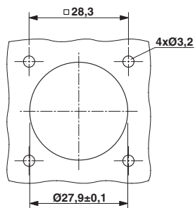
Maßzeichnung
