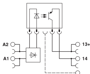
Schaltplan
