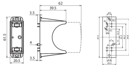
Maßbild DG PCB PV 500
