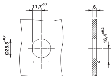
Maßzeichnung
