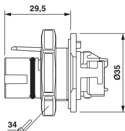
Maßzeichnung
