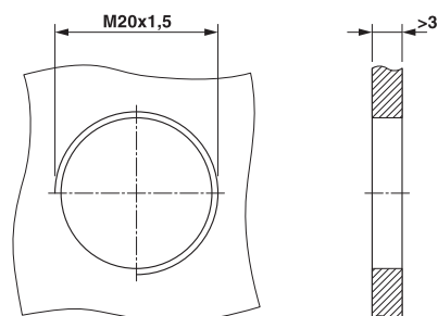
Maßzeichnung
