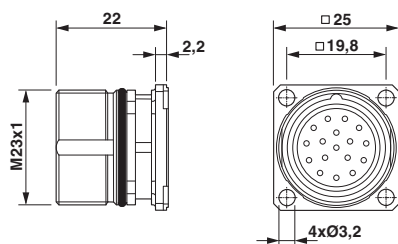
Maßzeichnung
