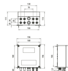
Maßbild DCU 2 YPV 1100 2M 1S MC4
