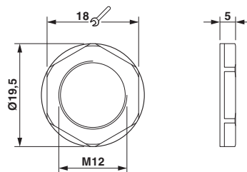
Maßzeichnung
