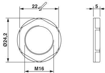
Maßzeichnung
