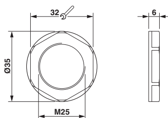
Maßzeichnung
