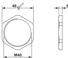
Maßzeichnung
