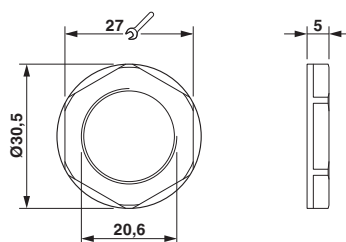
Maßzeichnung
