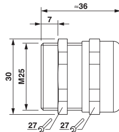
Maßzeichnung
