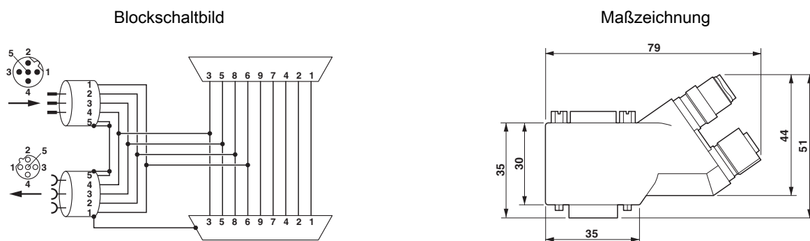
Funktionsschaltbild SUBCON-PLUS-PROFIB/...M12
