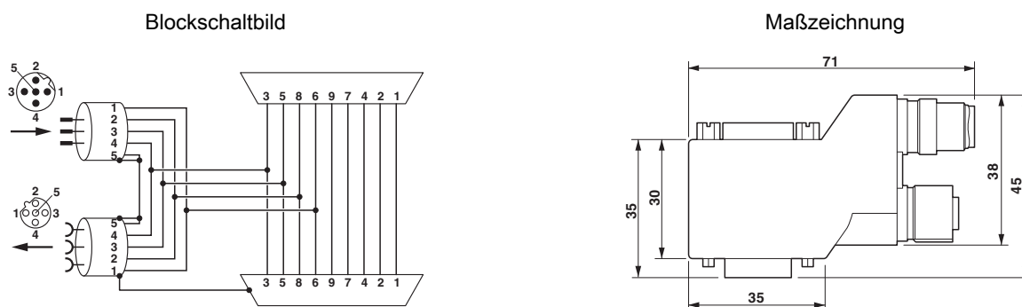
Funktionsschaltbild SUBCON-PLUS-PROFIB/...M12
