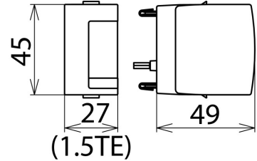
Maßbild DG MOD E DC 550
