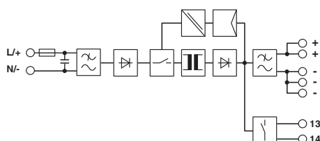
Blockschaltbild
