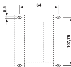
Maßzeichnung
