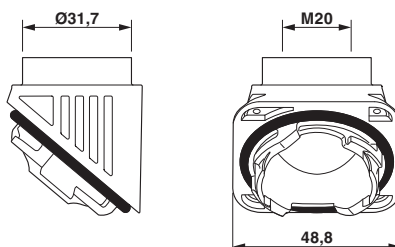
Maßzeichnung
