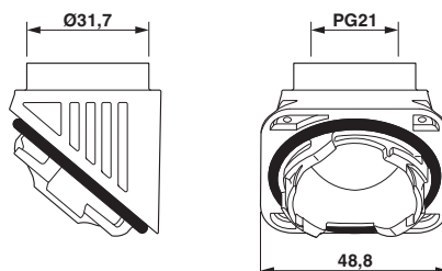
Maßzeichnung
