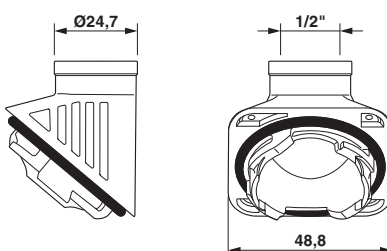
Maßzeichnung
