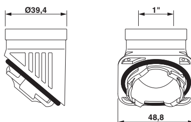
Maßzeichnung
