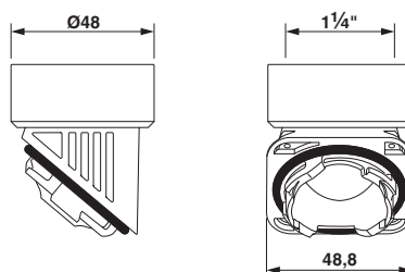
Maßzeichnung
