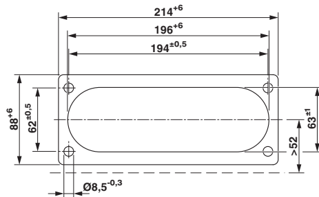
Wandausschnittszeichnung
