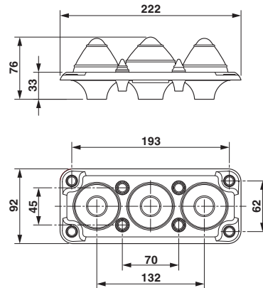
Maßzeichnung
